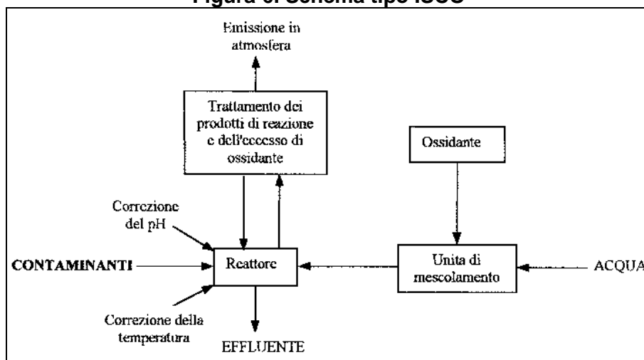
Figura 6. Schema tipo ISCO
