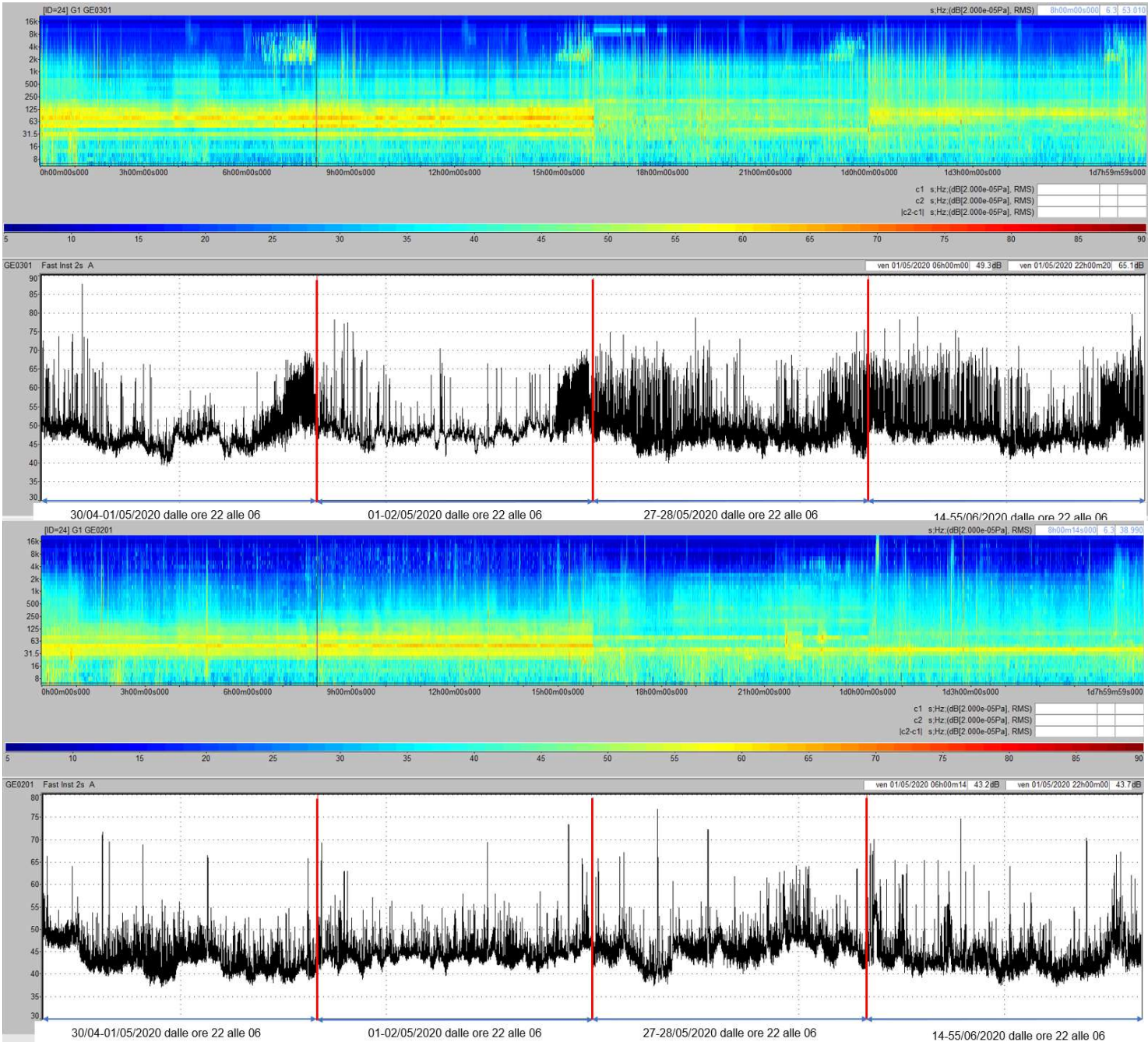
Figura 3: la sintesi del multispettro in banda 1/3 d'ottava di su 1 s in ponderazione lineare (dB) e dell'evoluzione temporale dei livelli LAeq su 1 s
