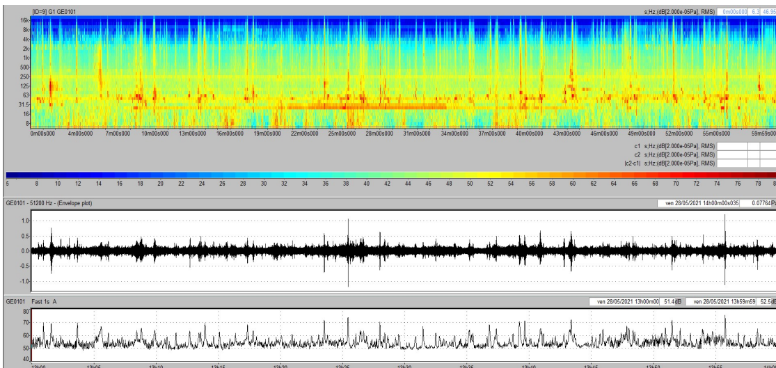
fréquence 1/3 octave 63Hz à 2 KHz (ligne verte) à proximité du site
