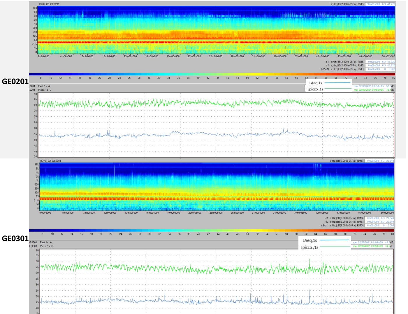
Figure 34: sonogrammes du Leq sur 1s (pondération linéaire, dB), niveau de Leq sur 1s (pondération A, dBA) et pic sur 1s (pondération C, dBC) pour la configuration de deux navires amarrés
