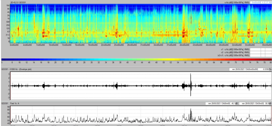
Figure 28: la synthèse du multispectre en bande 1/3 d'octave de sur 1 s en pondération linéaire (dB), de l'évolution du signal audio et de l'évolution temporelle des niveaux Leq sur 1s
