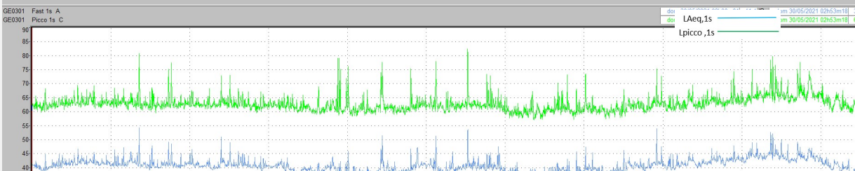
Figure 31: sonogrammes du Leq sur 1s (pondération linéaire, dB), niveau de Leq sur 1s (pondération A, dBA) et pic sur 1s (pondération C, dBC) pour la configuration d'un seul navire amarré
