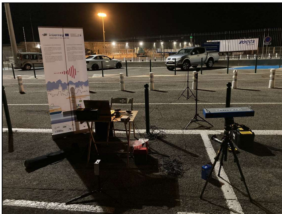
Figure24:Postation CPB en correspondance du tronçon 1
