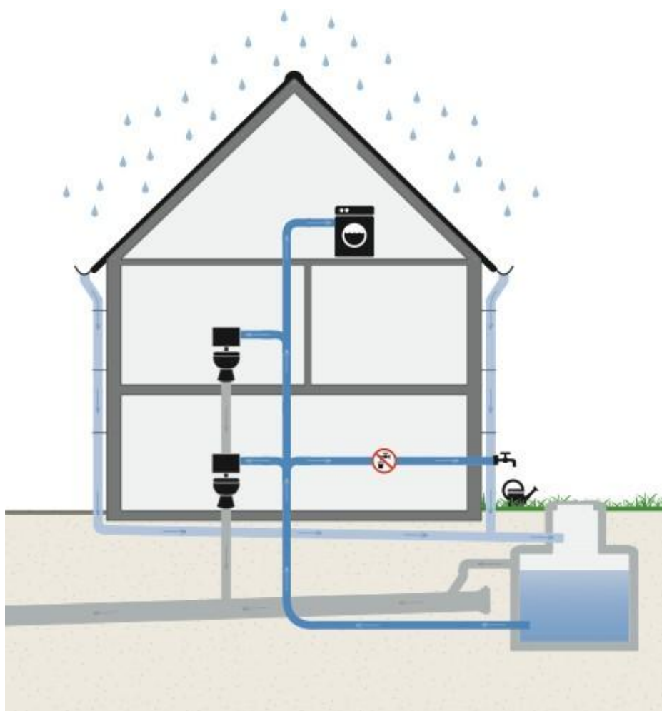
Fig. 4 – Sistema domestico per il recupero delle acque meteoriche
